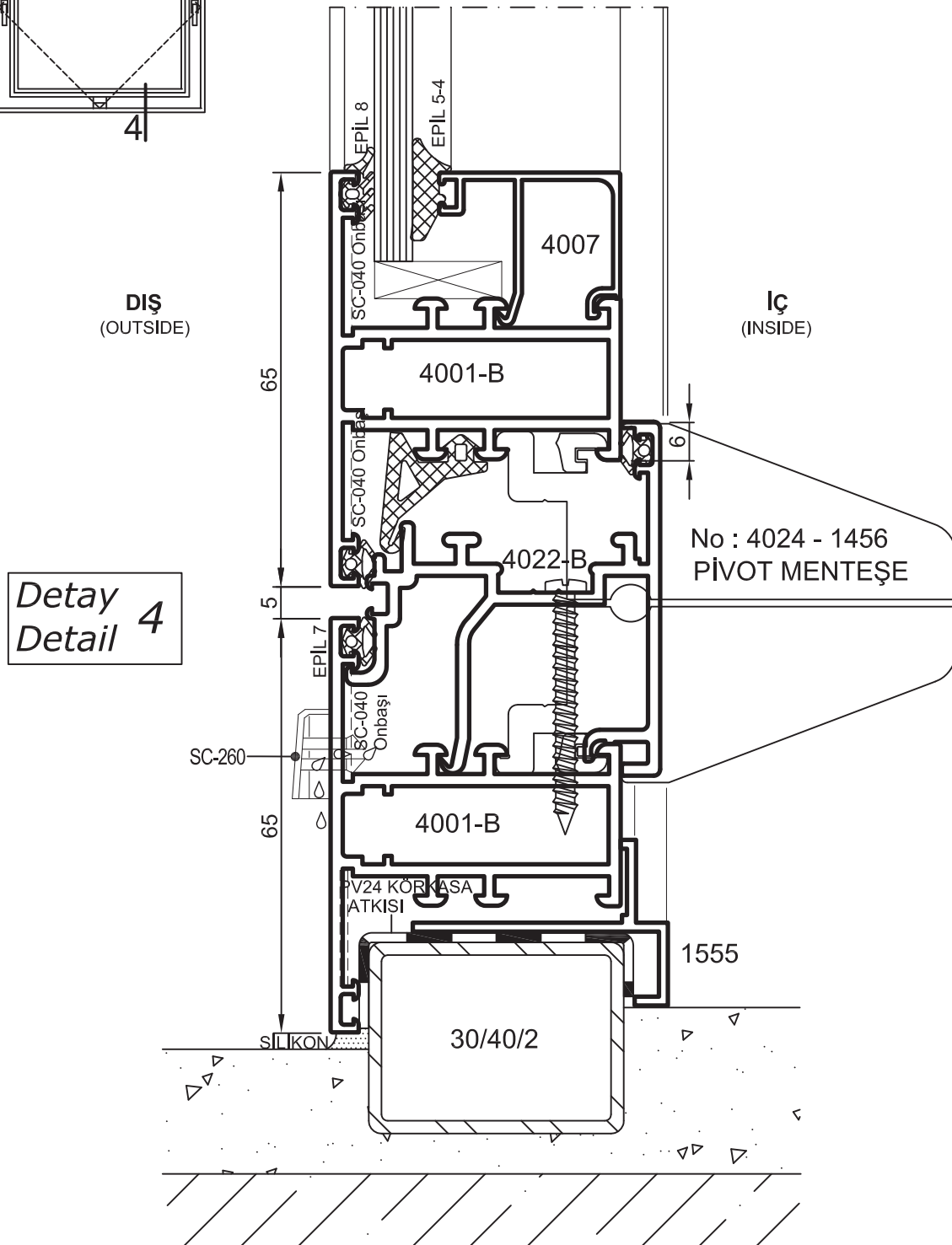
Pivot Window System Detail Pivot Pencere Sistem Detayı
