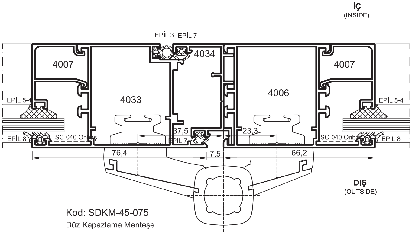
DIŞA AÇILIR KAPI DOOR - OUTSIDE OPENING
