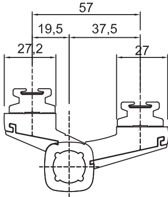
Kod: SFKM-45-070 Fugalı Kapazlama Menteşe
