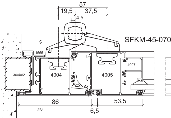
Kod: SFKM-45-070 Fugalı Kapazlama Menteşe
