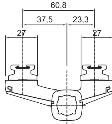
Kod: SDKM-45-075 Düz Kapazlama Menteşe
